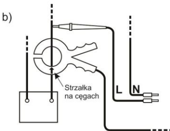
Sposób podłączenia cęgów
